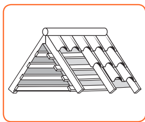
Тепло-, пароизоляция подкровельного пространства.
